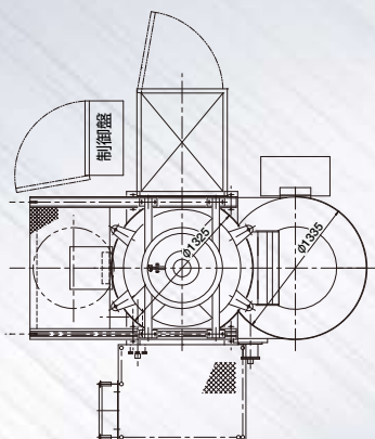
参考構成図 (MK-200型(L1))/Reference
